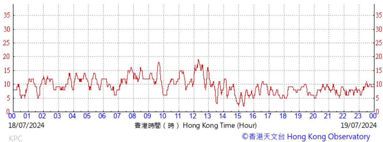
(公里/小時) (於香港時間19/07/2024 00時00分更新) (Updated at 00:00H on 19/07/2024) (km/h)
