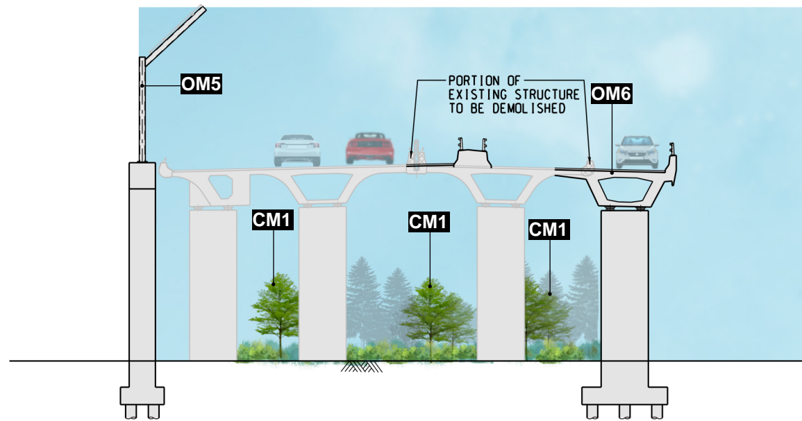
SECTION E - E
