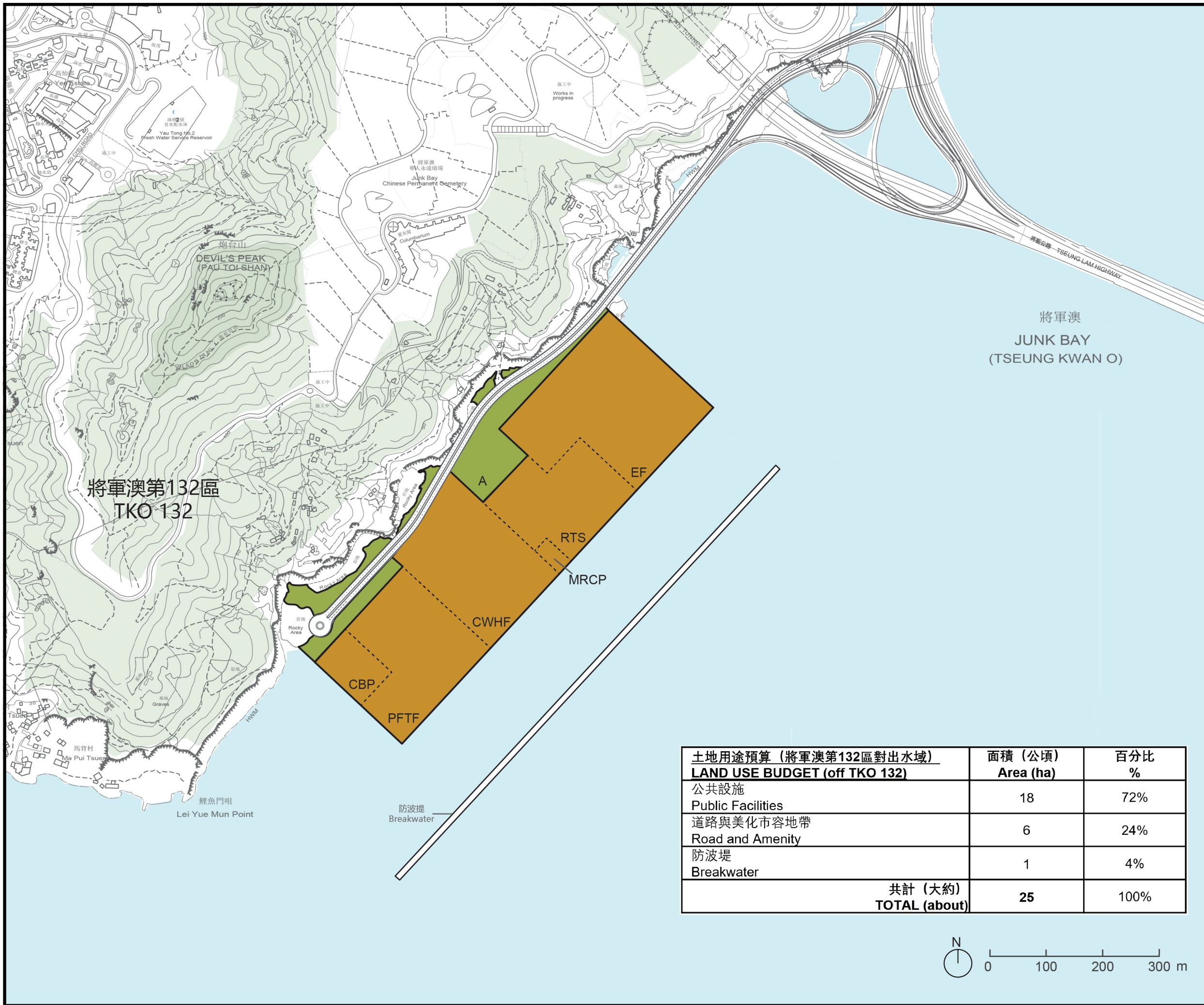
60720423/B30/FIGURE 2.7 將軍澳第132區對出水域範圍填海 初步發展大綱圖 Preliminary Outline Development Plan - Reclaimed land off TKO Area 132
